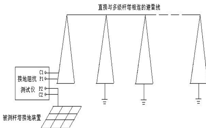
回路阻抗法测试杆塔接地阻抗示意图
