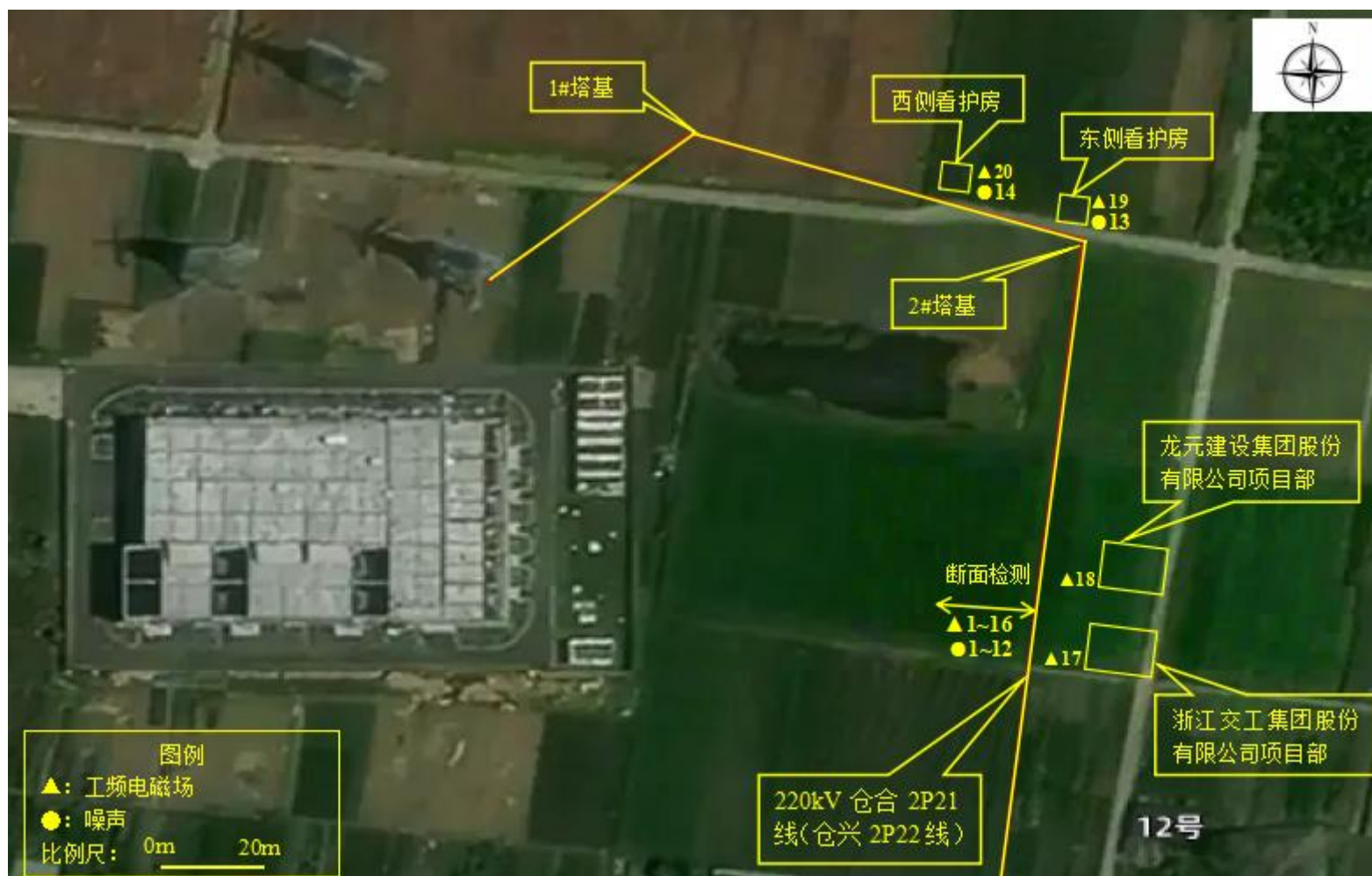
图 7-1 220kV 仓合 2P21 线（仓兴 2P22 线）2#-4#迁改工程工频电场强度、工频磁感应强度及噪声监测布点图
